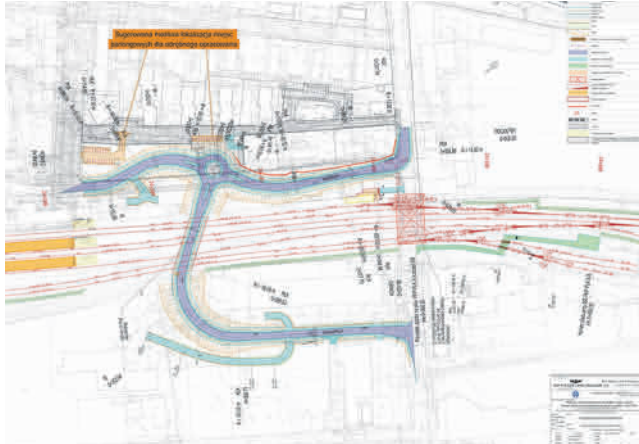
Zakres przebudowy i ingerencji w układ drogowy miasta przy budowie tunelu.
